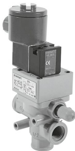
Bild 33: Magnetventil Typ 3962 Ex d (Ex em)
