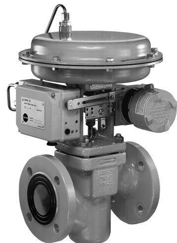
Bild 6: Stellungsregler Typ 4765/6116 Anbau an NAMUR-Rippe
