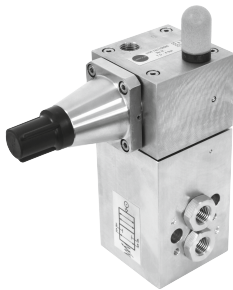
Bild 36: Pneumatisches Verblockrelais Typ 3709-5
